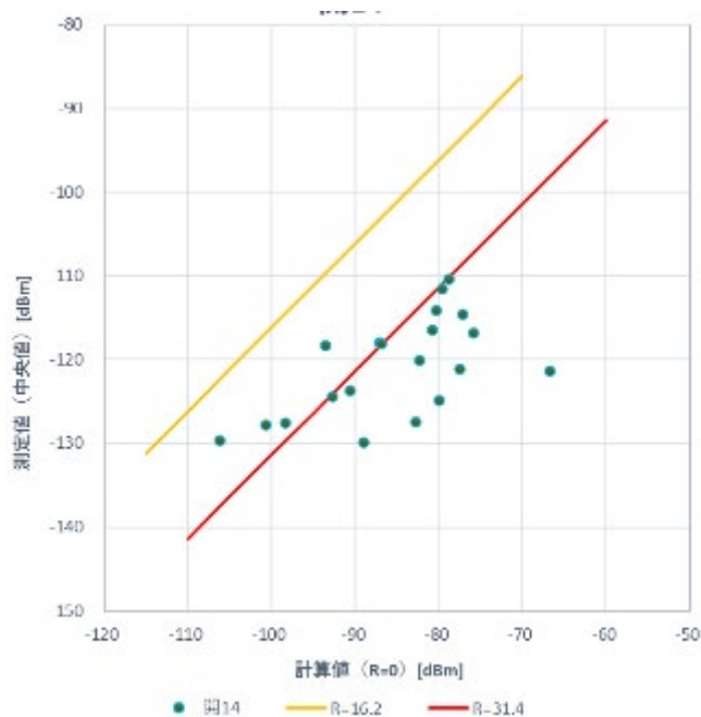
図 2. 2-8 中規模体育館での R 値の測定結果
