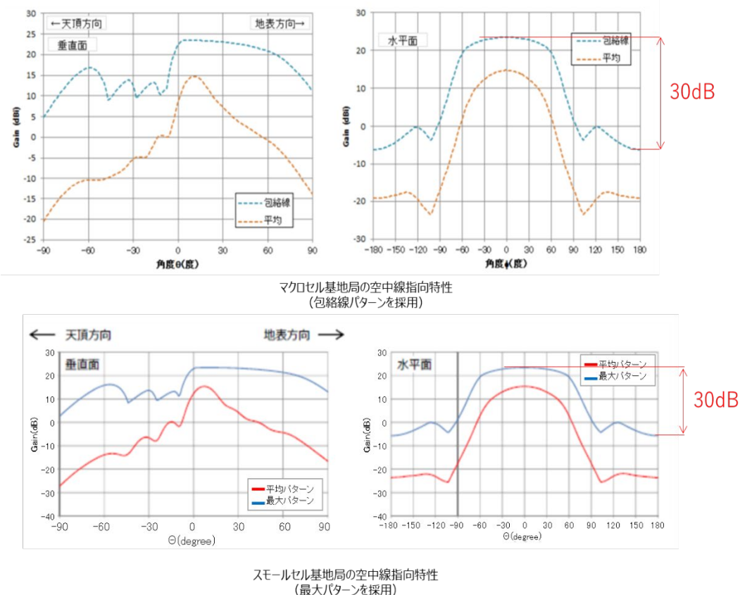
図 3. 3-1 受信電力 Pr 計算に用いた基地局空中線指向特性 (逆方向については 30dB 差があるとした)
