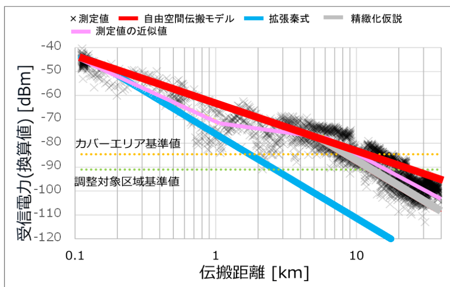
図 2. 2-13 海上における電波伝搬の測定結果
