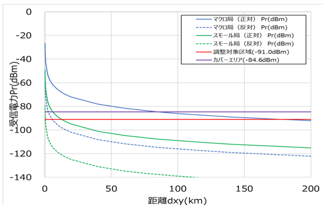
図 3. 3-3 同一周波数における受信レベル Pr
