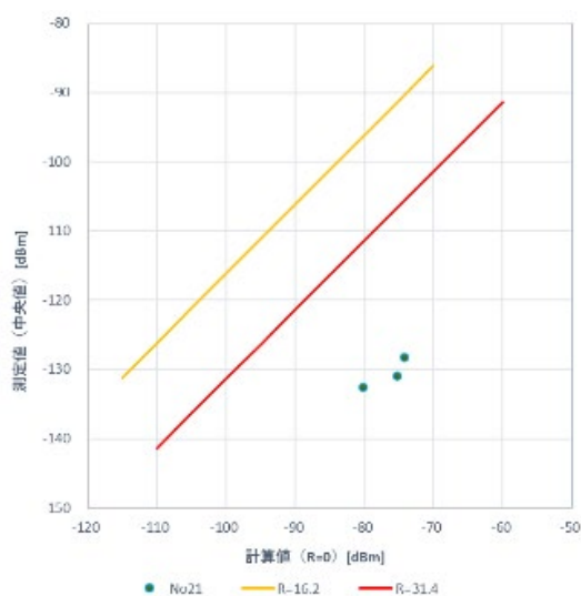
図 2. 2-4 コンサートホールでの R 値の測定結果
