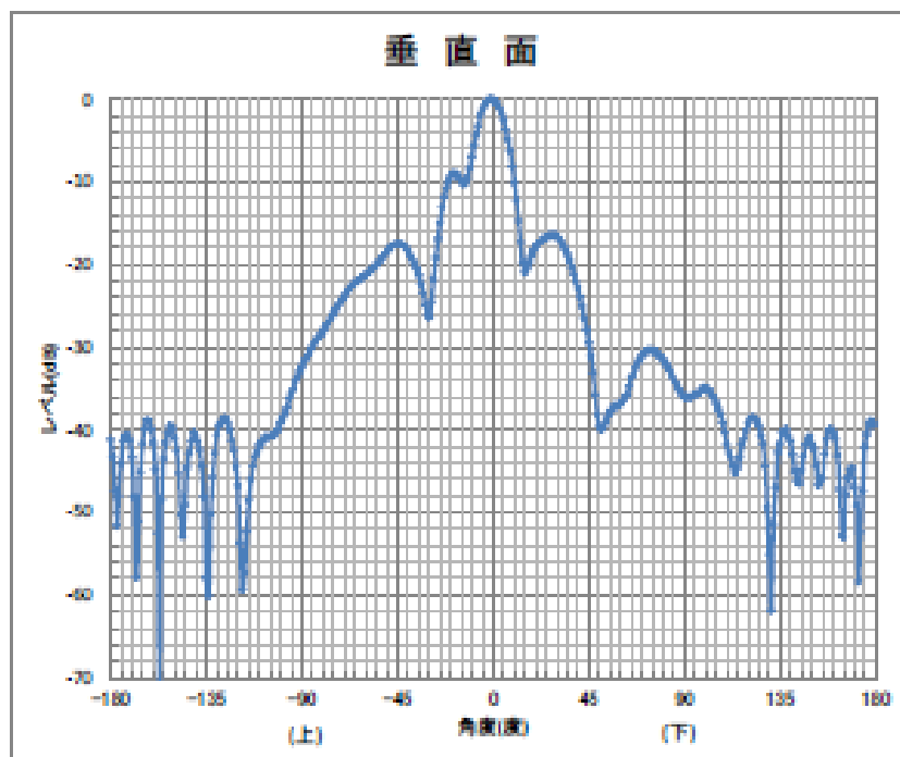
図 3. 2-15 5GHz 帯無線アクセスシステムの空中線指向特性
