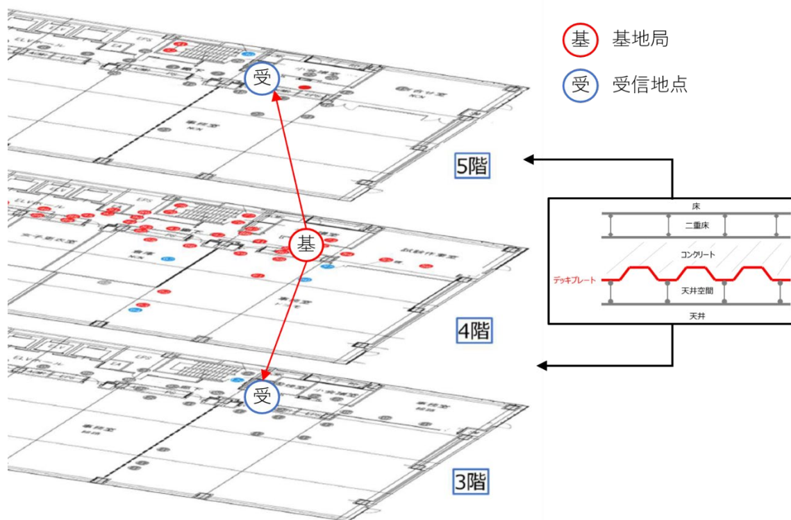
図 2. 2-9 階層を隔てた測定環境 (案件番号 R4-28)
