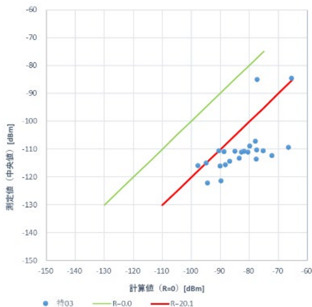
図 2. 2-12 地上駅ホームでのR値の測定結果
