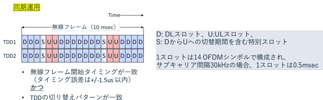
図 2. 2-14 同期運用
