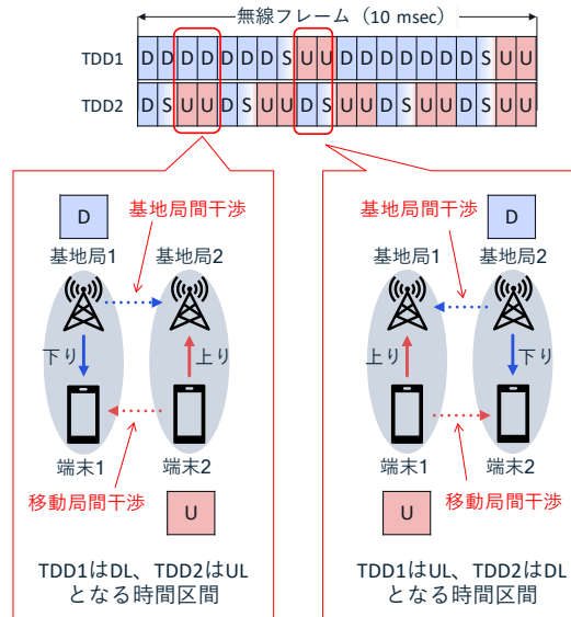
図 2. 2-16 非同期運用における基地局間・移動局間干渉
