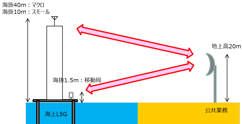
図 3. 2-5 今回の共用検討モデル (海上ローカル5Gシステムと公共業務)
